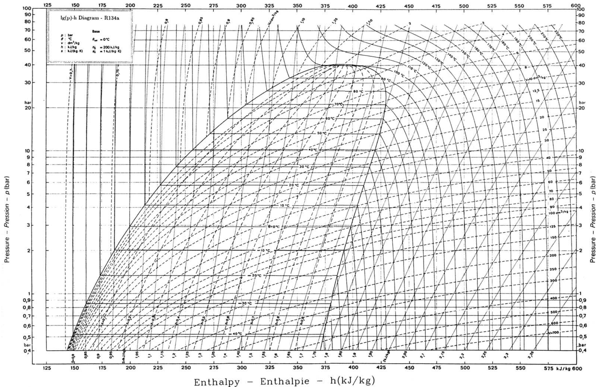
log p,h-Diagramm für R134a (C 2 H 2 F 4 )
